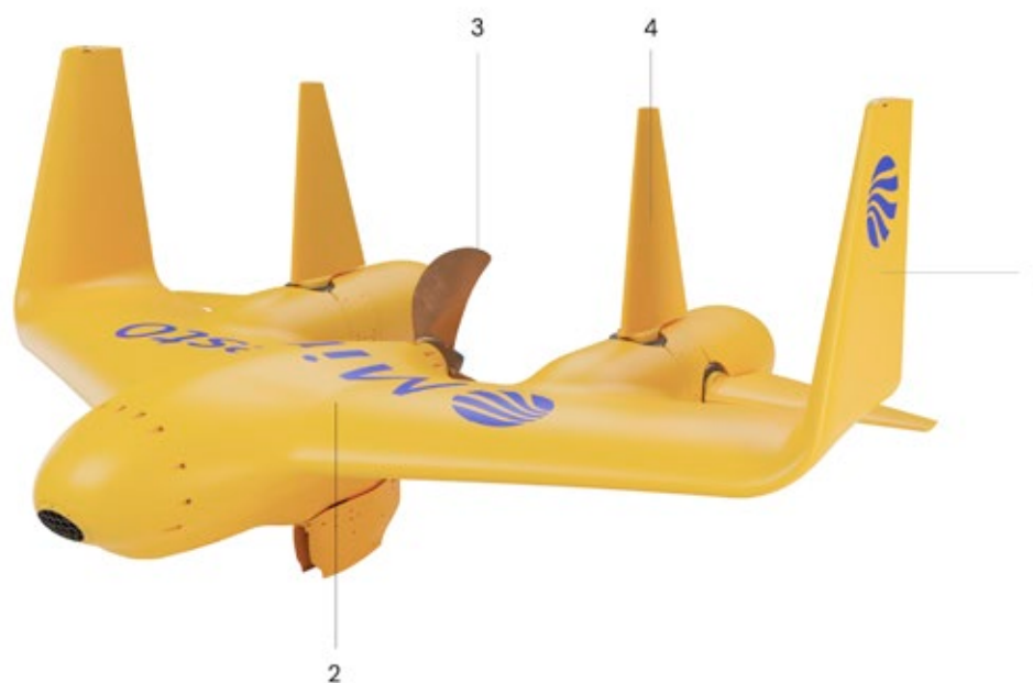
Bild 2. Minestos marina kraftverk består av en ving (1) som huserar ett maskinhus (2). Bakom vingen sitter turbinen (3), som är kopplad till en generator, och kraftverkets rodersystem (4). Rodersystemet styr kraftverket automatiskt i en förutbestämd bana. En förankringslina kopplar kraftverket till en förhöjningspunkt fäst i ett fundament på havsbotten. Förankringslinan rymmer elkablar såväl som kablar för kommunikation. Källa: Minesto
