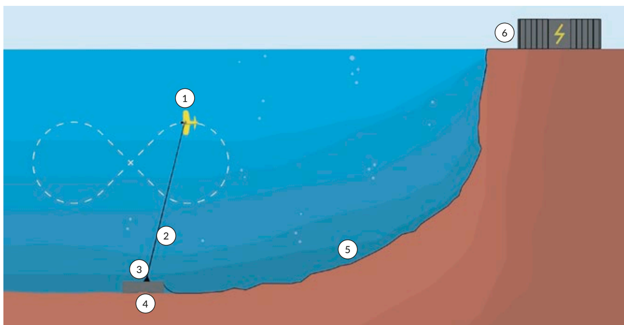
Bild 1. Illustration över de olika delarna vid en installationsplats för Minestos teknik vilka är 1) Kraftverk som genererar elektricitet, 2) Förankringslina som kopplar ihop kraftverket med bottenförankringen, 3) Bottenförankringen som är kraftverkets "svängpunkt", 4) Fundament på havsbotten, 5) Sjökabel för kraftöverföring samt datakommunikation och 6) Anslutningspunkt till elnät på land eller till annan användning. Källa: Minesto
