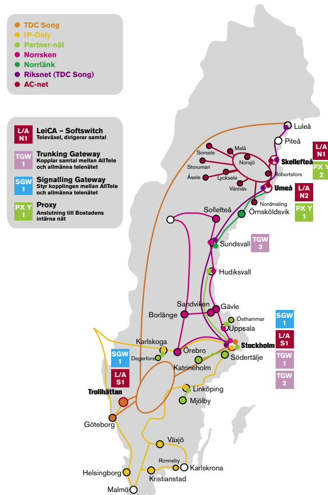
Figur 1. Schematisk översikt av AllTeles växel- samt överlämningspunkter mellan Bolagets samarbetspartners olika fiberoptiska nät, stadsnäten och det äldre allmänna kopparbaserade telefoninätet (PSTN)
