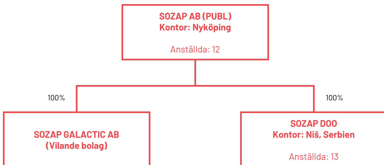
Figur 8: Koncernstruktur
