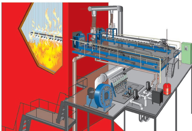
Ecotube-systemets olika delar
