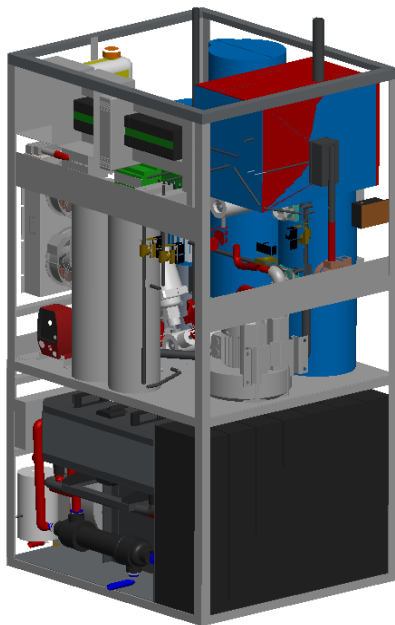
Bilden visar 3D CAD modell och seriedesign för 5 kW kraftvärmesystem "Prometheus 5"
