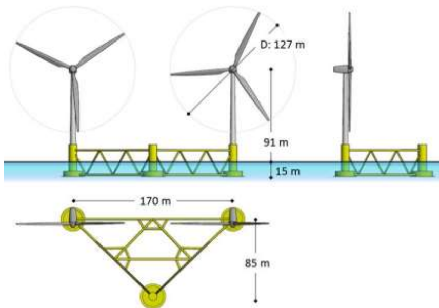
Figur 2: Illustration av plattformen med ungefärliga dimensioner
