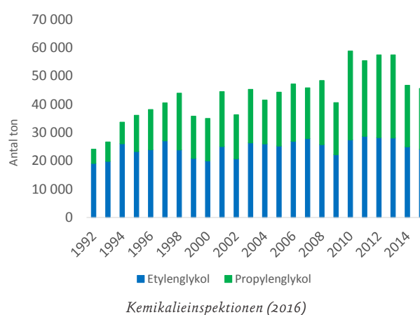
Antal ton importerad och tillverkad glykol i Sverige 1992-2015
