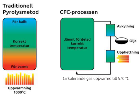
Enviros process i jämförelse med traditionell pyrolys.
