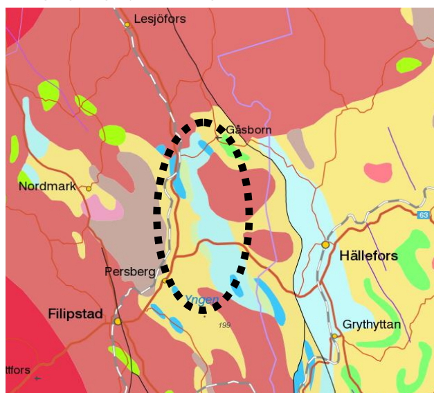
Berggrundskarta över Saxå-objektet
